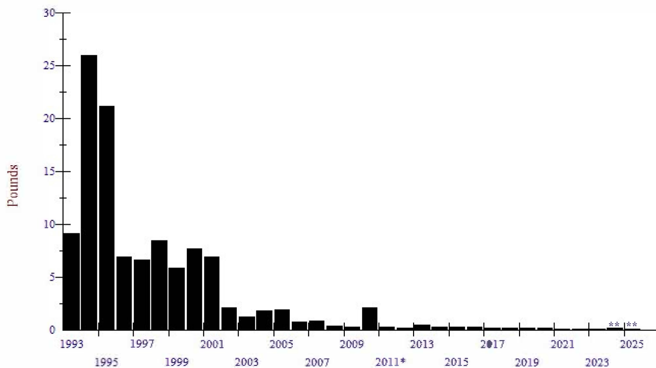
Bucklin Point Effluent Mercury Loading
